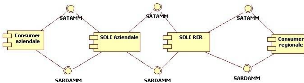
Figura 2: Relazione logica tra i sistemi
